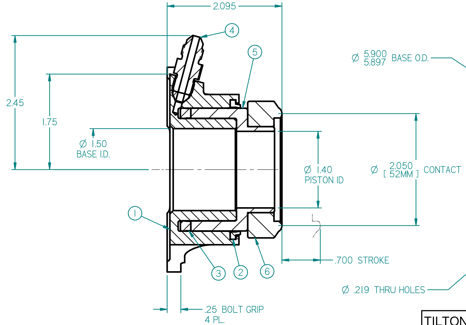
SECTION A-A
