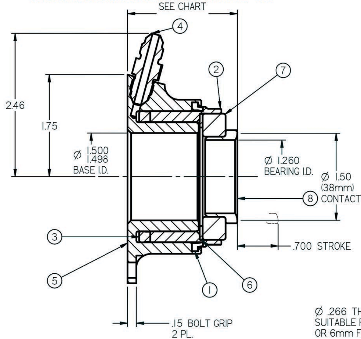
SECTION A-A
